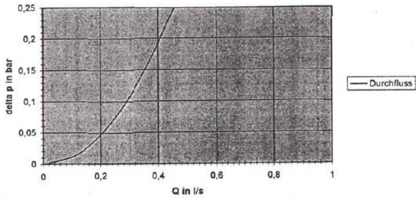
Durchfluss-Diagramm Schmutzfänger
