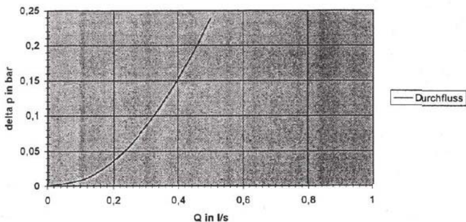
Durchfluss-Diagramm Schmutzfänger
