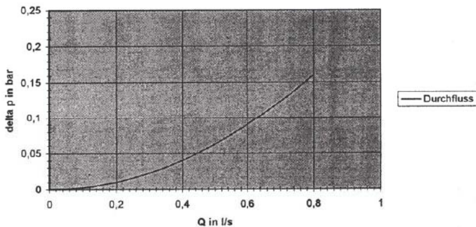
Durchfluss-Diagramm Schmutzfänger
